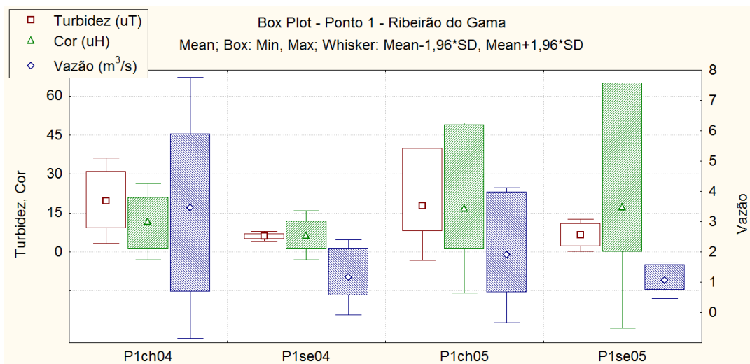
Figura 45 – Comportamento da turbidez e cor nos períodos chuvosos e secos. Ponto 1.
