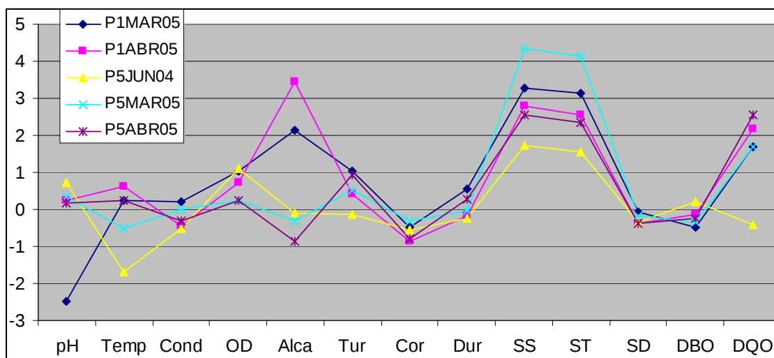
Figura 70 – Gráfico resultante da padronização das observações do Grupo 2 no Ribeirão do Gama.
