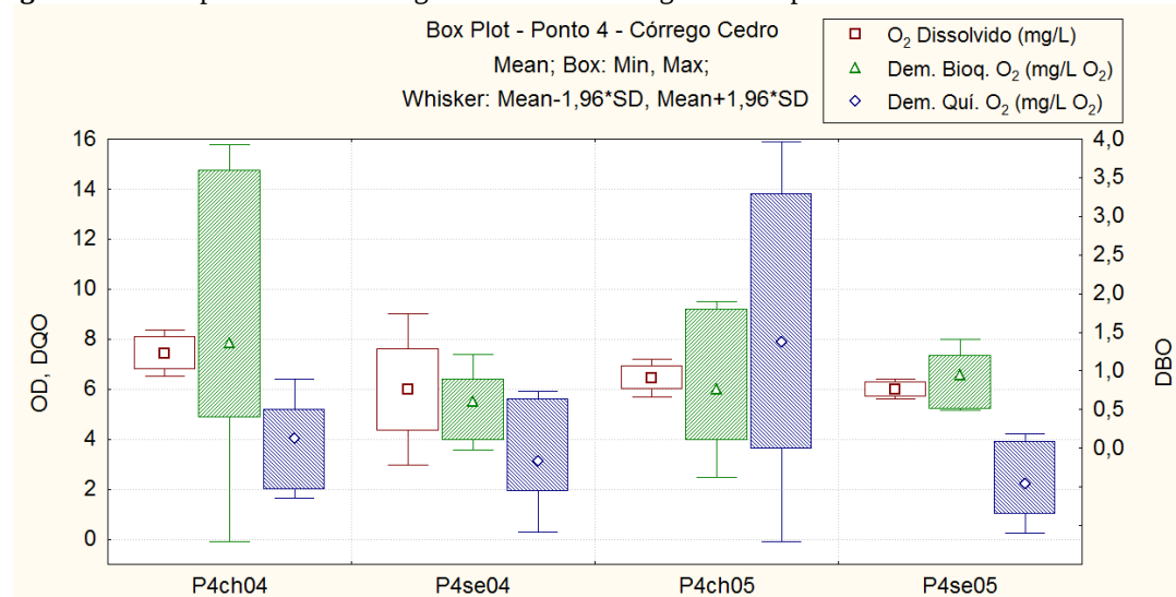
Figura 59 – Comportamento do oxigênio e da matéria orgânica nos períodos chuvosos e secos. Ponto 4.
