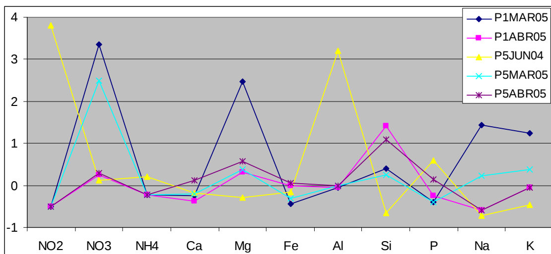
Figura 71 – Gráfico resultante da padronização das observações do Grupo 2 no Ribeirão do Gama.
