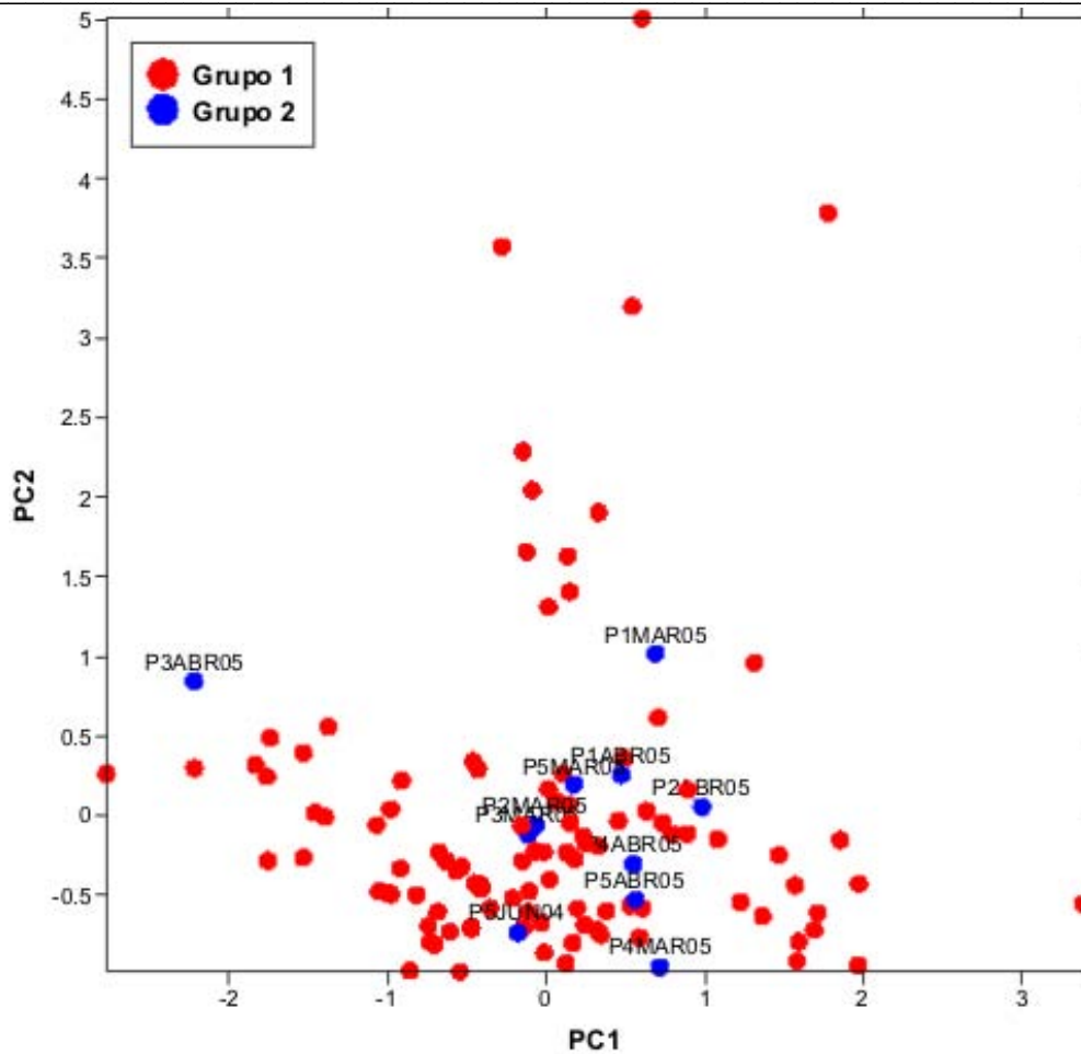
Figura 65 – Gráfico de espalhamento dos pesos das observações nas duas primeiras principais componentes. As observações nomeadas são as que diferem do padrão normal, segundo o método k-médias de agrupamento.
