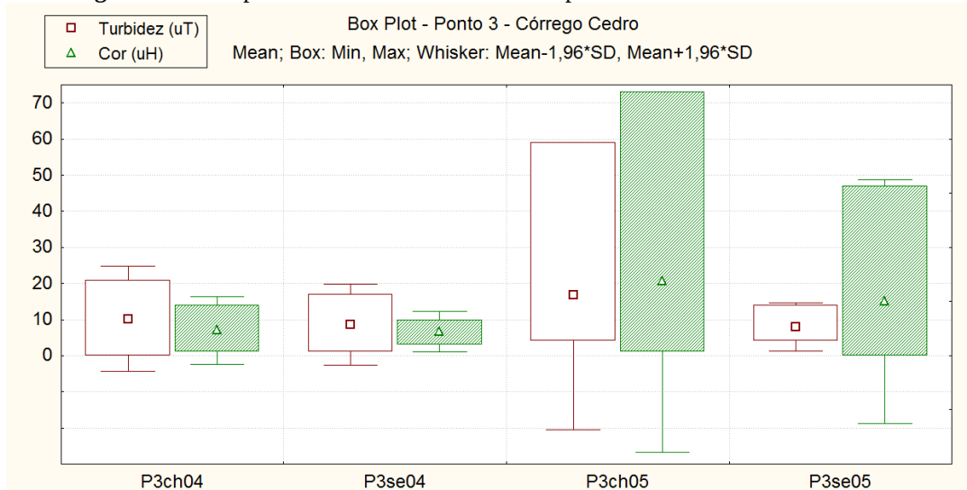
Figura 43 – Comportamento da turbidez e cor nos períodos chuvosos e secos. Ponto 3.
