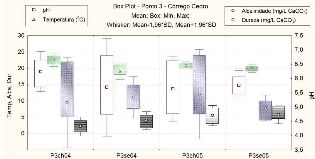
Figura 38 – Comportamento de parâmetros físico-químicos nos períodos chuvosos e secos. Ponto 3.
