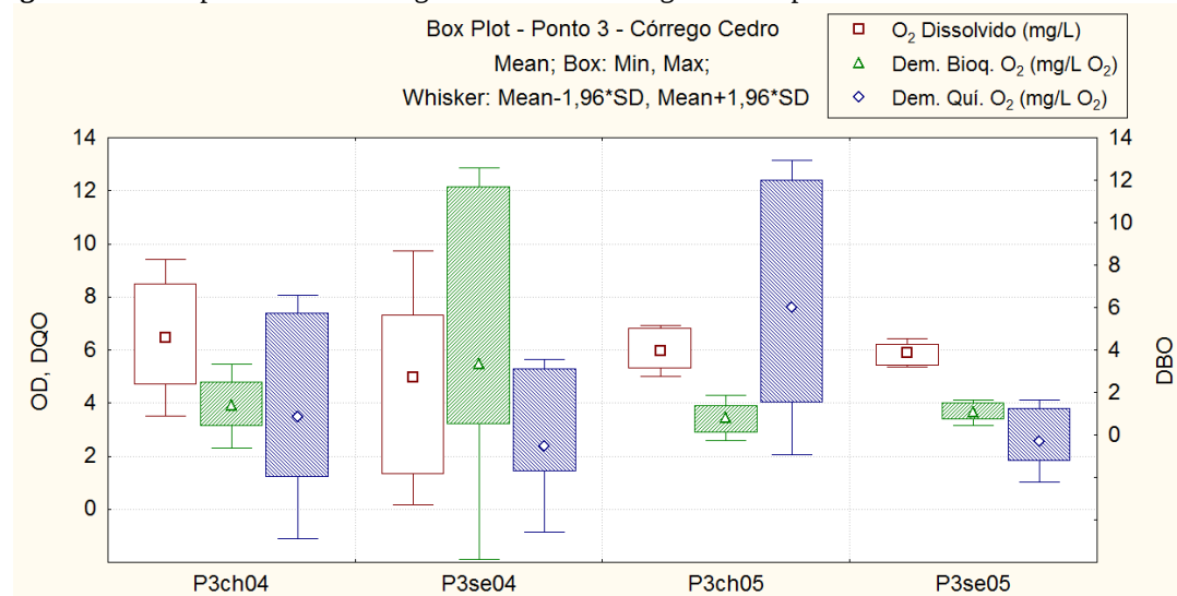
Figura 58 – Comportamento do oxigênio e da matéria orgânica nos períodos chuvosos e secos. Ponto 3.
