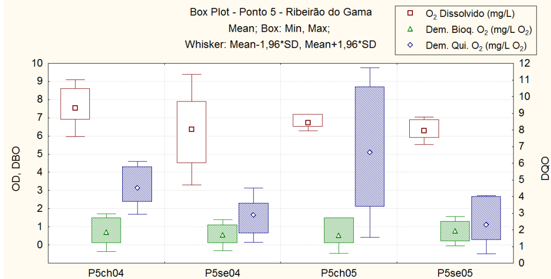
Figura 61 – Comportamento do oxigênio e da matéria orgânica nos períodos chuvosos e secos. Ponto 5.
