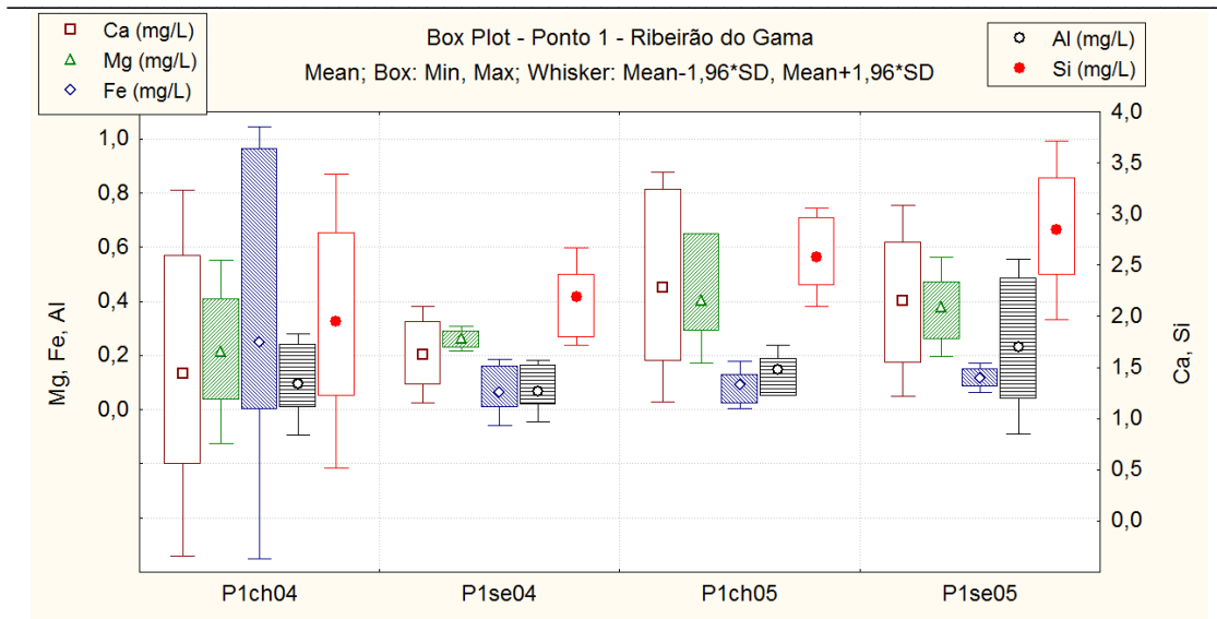
Figura 26 – Comportamento do Ca, Mg, Fe, Al e Si nos períodos chuvosos e secos. Ponto 1.
